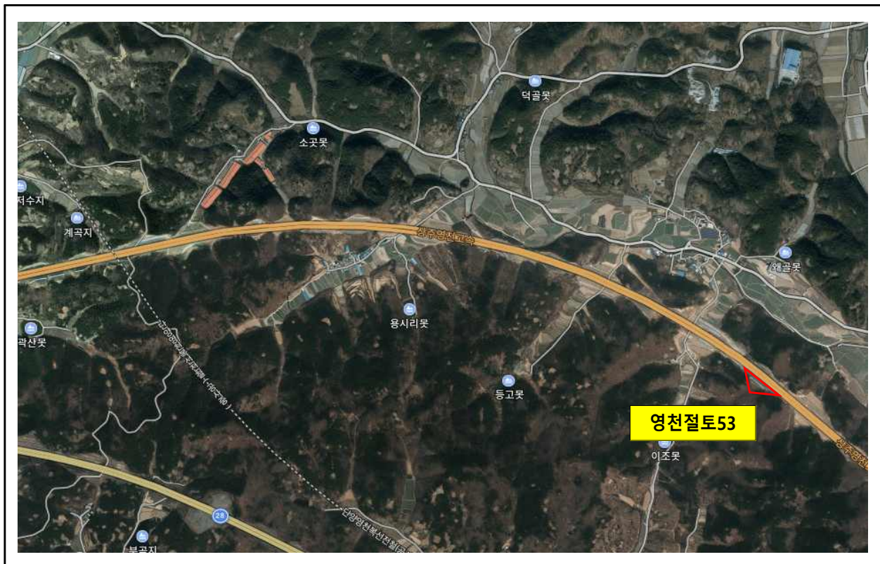
【그림 53.13】 영천절토53 검토대상 비탈면구간
