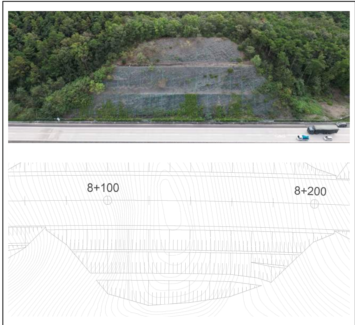
【그림 53.14】 영천절토53 검토대상 비탈면구간
