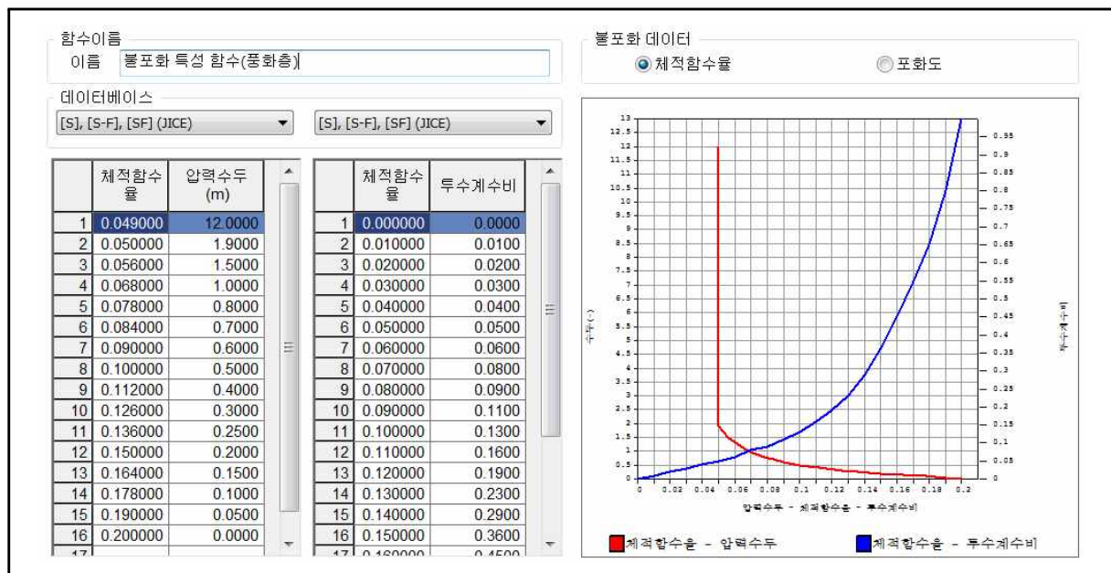
【그림 53.15】 압력수두-체적함수율(포화도)-투수계수비 함수
